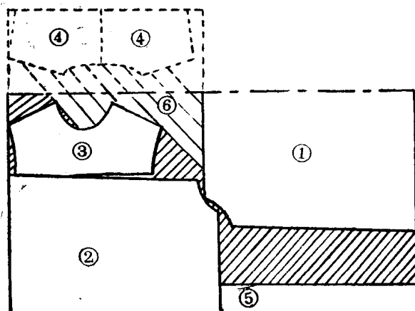
女童春秋上衣排料图
