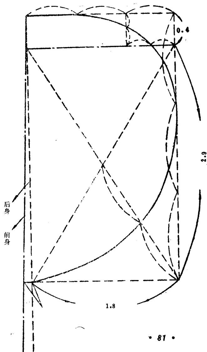
领口实线图
