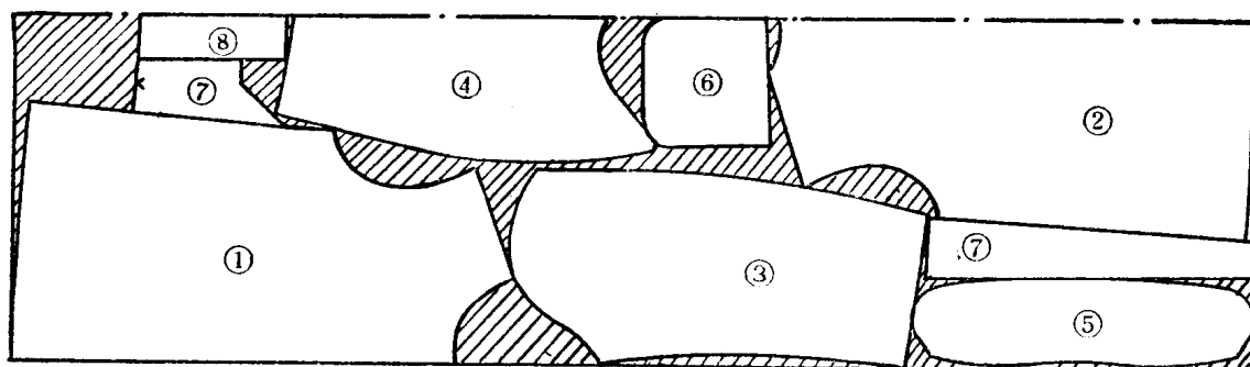
女童长袖衬衣排料图
